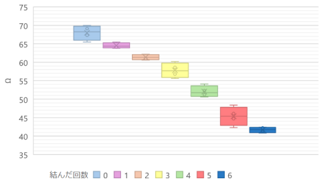
図 10 結んだ回数による抵抗値の変化
