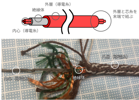
図 7 2層組紐の構造と制作例
