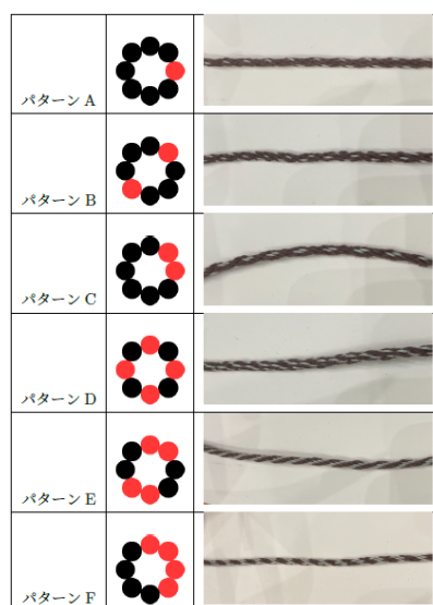
図 5 制作した導電組紐。模式図の赤が導電糸の配置箇所
