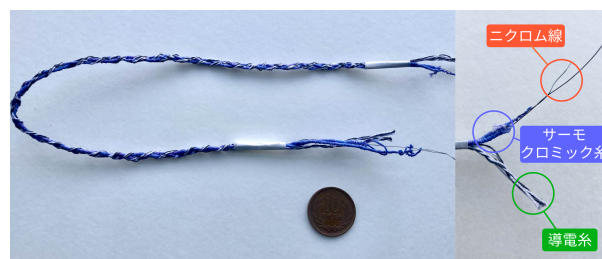
図 18 導電糸とサーモクロミック糸を組み込んだ組紐
