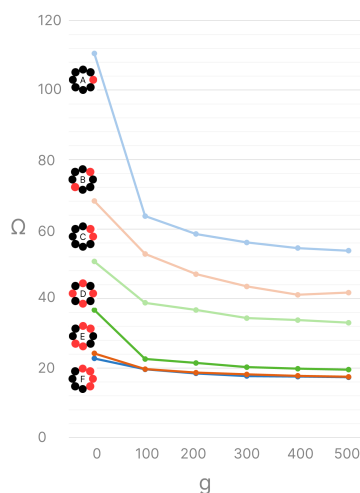
図 6 引張による抵抗値の変化
