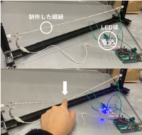
図 11 制作事例：引張に応じて光量が変化する
